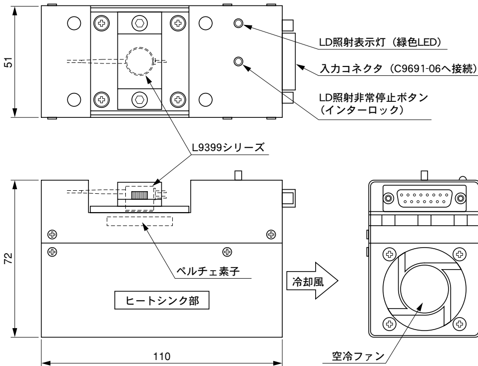
図1 外形寸法図 (単位: mm)
