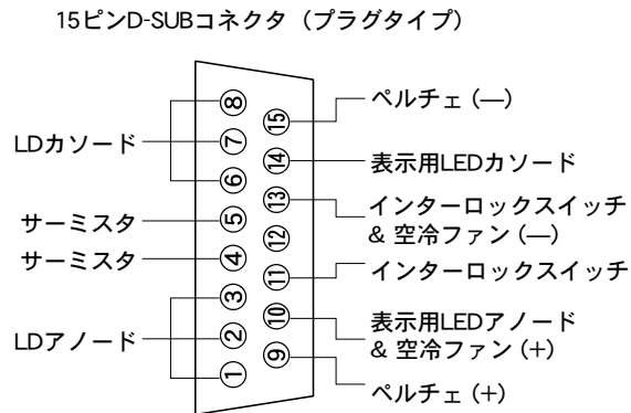
図2 入力コネクタ接続図
