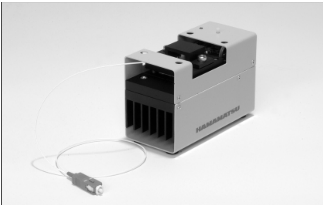
ファイバ出力型LD L9399-02をマウントしたC10096-01 外観 (L9399-02は、別売りです。)
